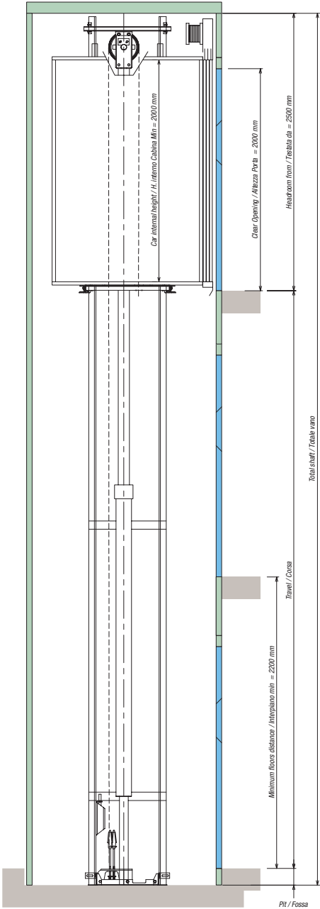
Tower shaft - vertical section Vano incastellatura - sezione verticale
