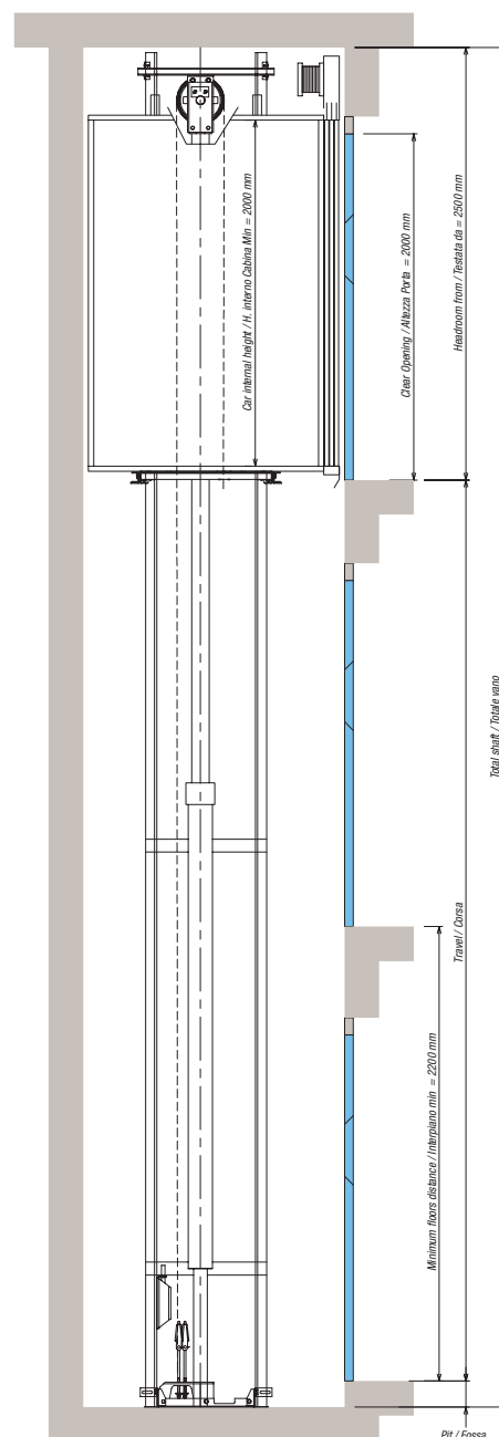
Shaft in bricks-vertical section Vano in muratura - sezione verticale
